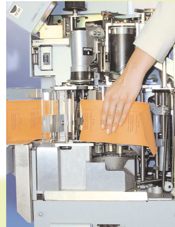
Einfaches Einlegen der Papierrolle für die Münzverpackung (Abb. links). Ein wesentliches Prinzip der gesamten NGZ-Technologie: klar verständliche Angaben auf den Bedienungs-Displays (Abb. rechts).
